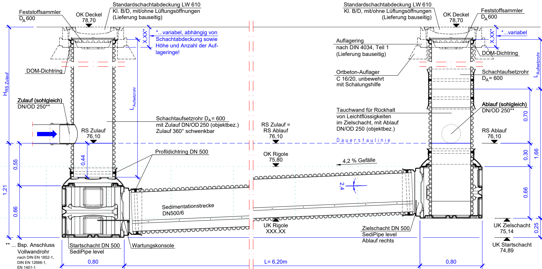
Regenwasserbehandlung nach DWA-M 153 SediPipe level 500/6, Ablauf rechts
